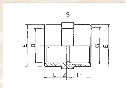
PVC Mufna připojení – lepení x závit int. barva – šedá (int. = vnitřní)
