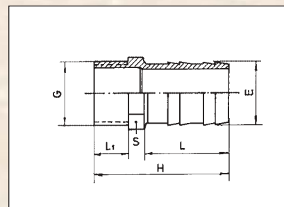
PVC Trn hadicový připojení – závit ext. barva – šedá (ext – vnější)
