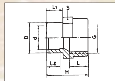
PVC Mufna – přechodka redukovaná připojení – lepení x závit int. barva – šedá (int. = vnitřní)
