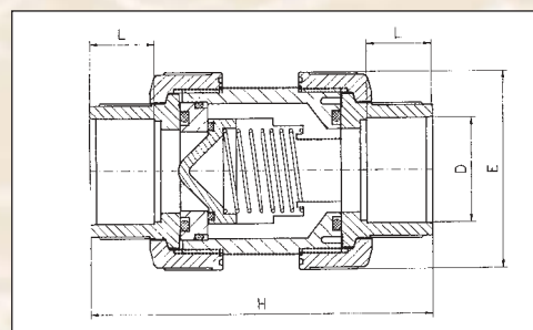
PVC Kuželový zpětný ventil připojení – lepení barva – šedá
