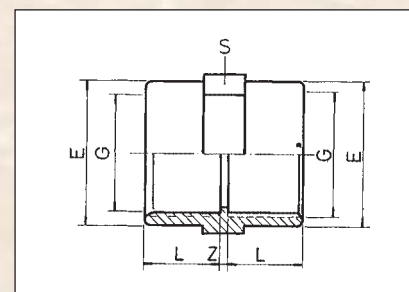
PVC Mufna připojení – závit int. x závit int. barva – šedá (int. = vnitřní)
