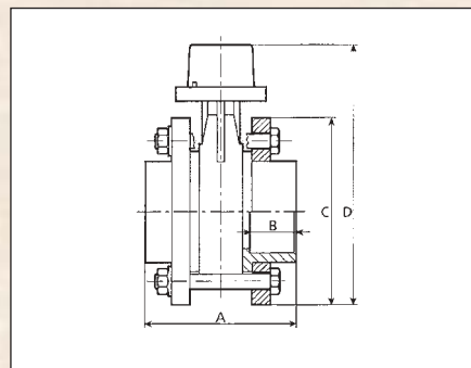
Uzavírací klapka (s přírubou a manžetou) těsnění EPDM
