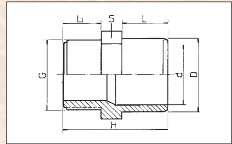
PVC Mufna – přechodka připojení – lepení x závit ext. barva – šedá (ext. = vnější)
