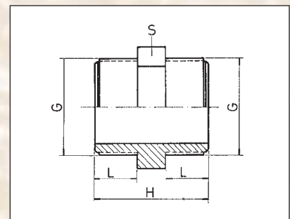
PVC Dvojnipel připojení – závit ext. x závit ext. barva – šedá (ext. = vnější)
