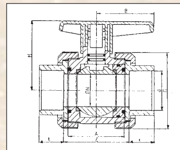
PVC Kulový dvoucestný ventil připojení – lepení barva – šedá
