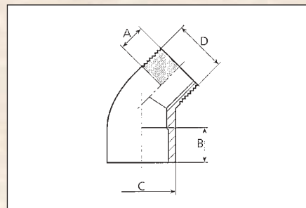
PVC Úhel 45° připojení – lepení x závit ext. barva – šedá (ext. – vnější)
