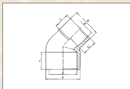
PVC Úhel 45° připojení – lepení int. x lepení ext. barva – šedá (ext. – vnější), (int. – vnitřní)
