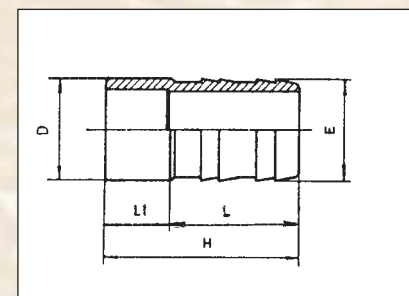
PVC Trn hadicový připojení – lepení barva – šedá
