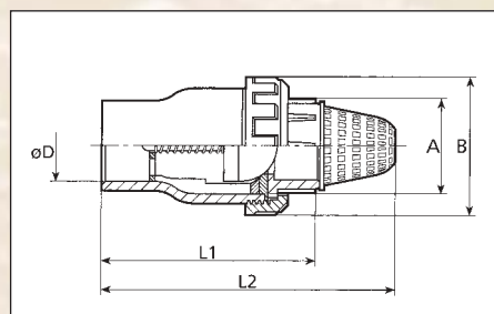
PVC Kuželový zpětný ventil s košem připojení – lepení barva – šedá
