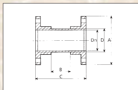
Průhled s přírubami PN-10
