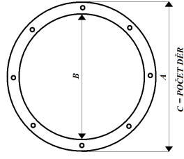
1. MTS Č.z. 3653 - sada A – 10,6 cm B – 7,1 cm C – 6 ks Těsnění : E355302 Rámeček : 36532
