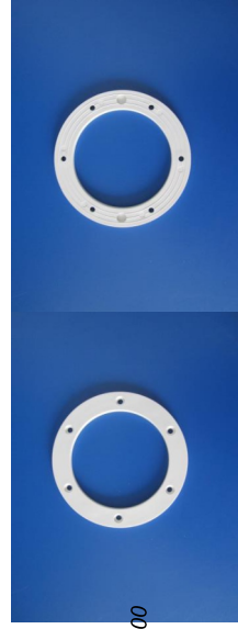
4. KRIPSOL - Podlahová Č.z. – KR85107890 A – 14,9 cm B – 10,7 cm C – 6 ks Těsnění : KR85107900
