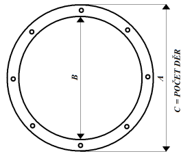
5. COFIES 35/50/75W Č.z. – HPRH20029 A – 12 cm B – 8,2 cm C – 6 ks Těsnění : HPRH20030 Rámeček : HPRH7009
